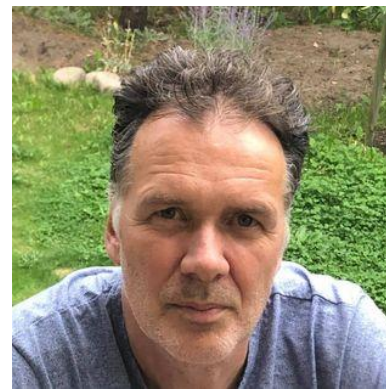
😊 LUFCMOT 😊
